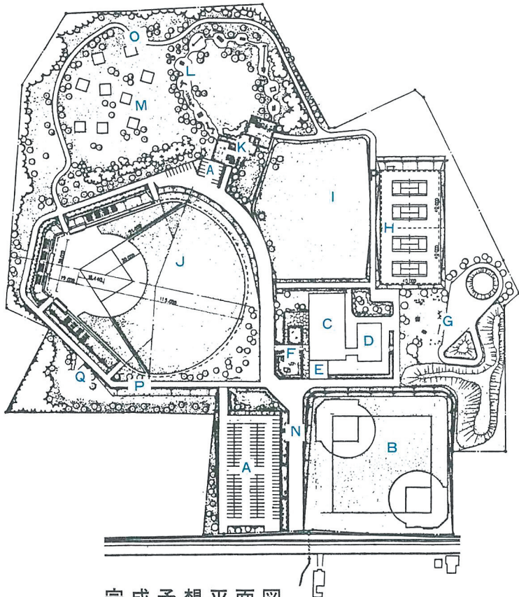
完成予想平面図
